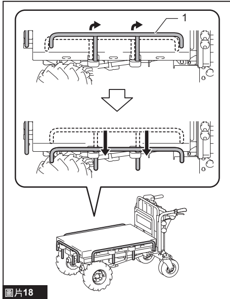
► 1. 防護架
