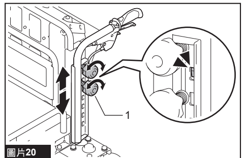
► 1. 旋鈕
