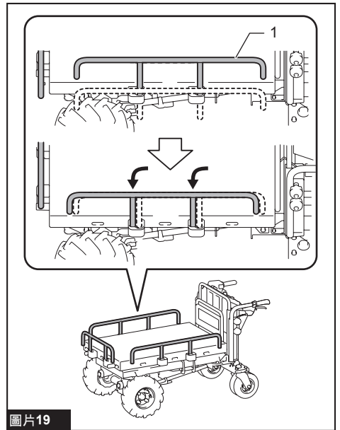
► 1. 防護架
