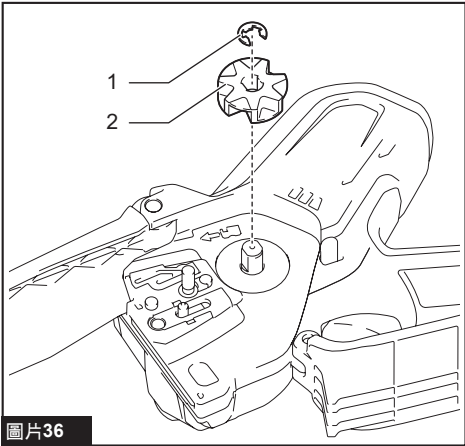
► 1. 鎖定環 2. 鏈輪
