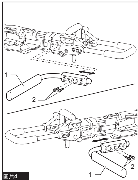
► 1. 反作用力接收器桿 2. 螺栓 C
