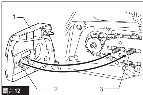
圖片12 ► 1. 鏈輪護蓋 2. 開孔 3. 螺栓
