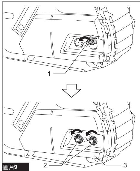
圖片9 ► 1. 鏈條調整螺絲 2. 固定螺帽 3. 鏈輪護蓋
