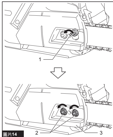
► 1. 鏈條調整螺絲 2. 固定螺帽 3. 鏈輪護蓋
