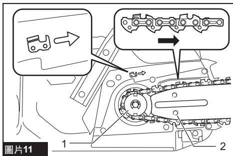
圖片11 ► 1. 鏈輪 2. 開孔
