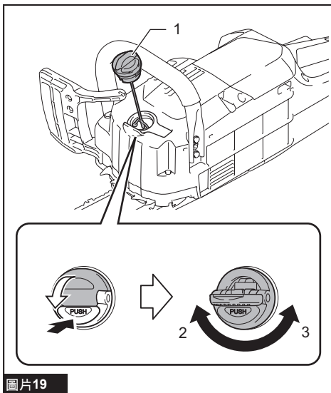
► 1. 油箱蓋 2. 鎖緊 3. 鬆開
