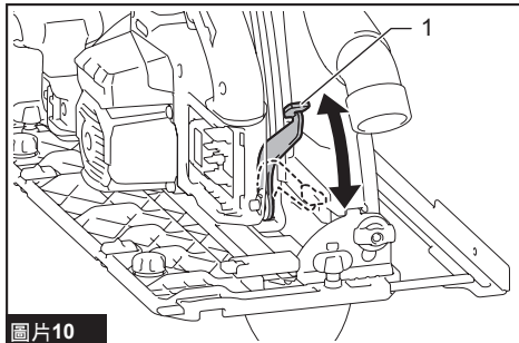
► 1. 鎖定桿
