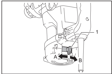
▶ 1. 反轉開關桿
