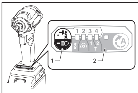
▶ 1. 按鈕 2. 開關面板
