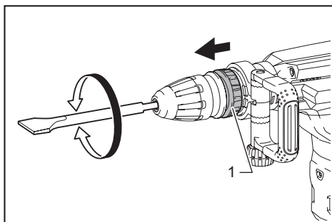
► 1. 切換環蓋
