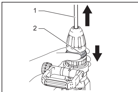
► 1. 鑽頭 2. 釋放蓋
