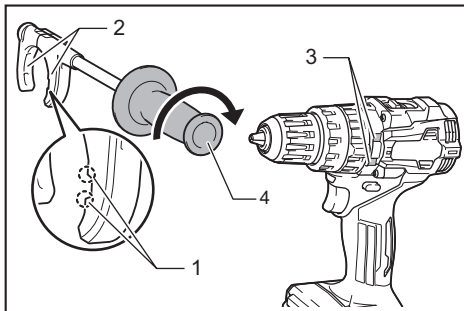
► 1. 凸起部分 2. 支臂 3. 凹槽 4. 把手
