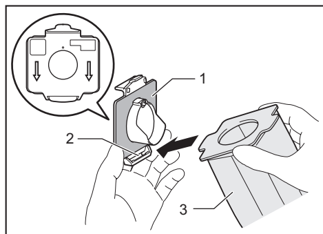
► 1. 防塵擋板 2. 溝槽 3. 濾紙
