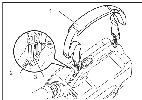
► 1. 肩帶 2. 鉤環 3. 安裝座
