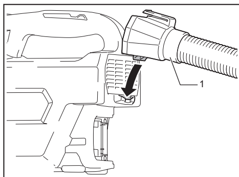
► 1. 吹風機組件
