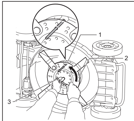
► 1. 插銷 2. 基板 3. 套筒扳手
