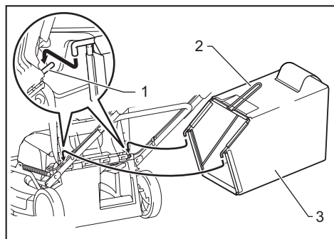
► 1. 桿 2. 把手 3. 草籃
