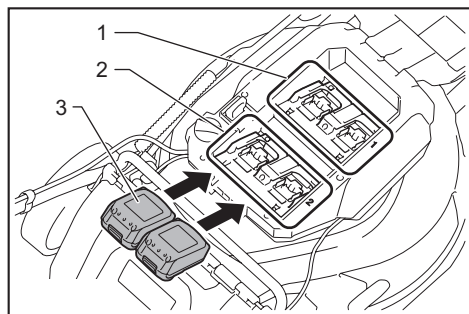
► (1) 電池埠 (2) 電池埠 (3) 電池組
