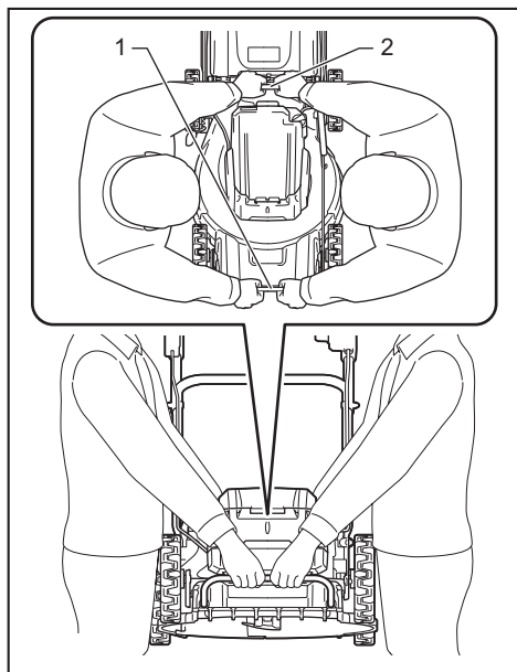
► 1. 前把手 2. 後把手
