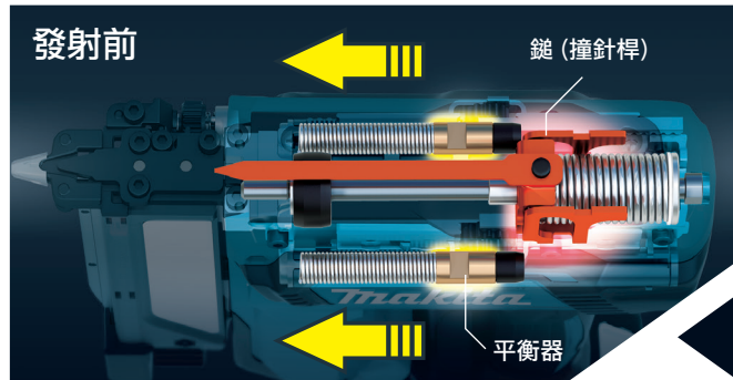
發射前 當活塞向後退時，平衡器會往前
