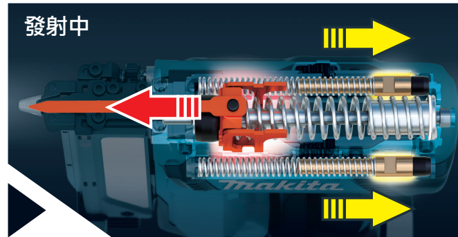
發射中 此設計能減少反作用力
