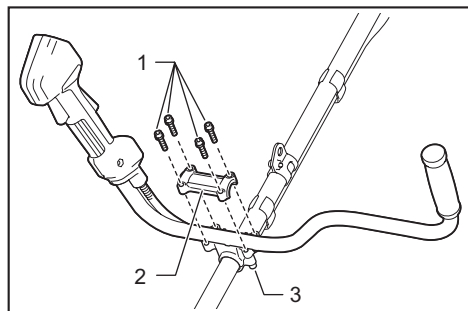
► 1. 內六角螺栓 2. 把手固定夾 3. 把手固定座
