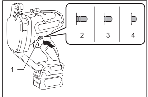
▶ 1. 反轉開關桿 2. 切割位置 3. 鎖定位置 4. 反轉位置
