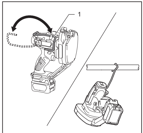
► 1. 固定鈎
