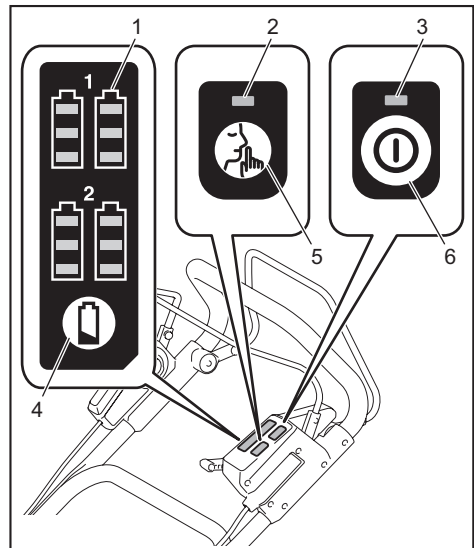
► 1. 電池指示燈 2. 模式切換燈 3. 主電源指示燈 4. 檢查按鈕 5. 模式切換按鈕 6. 電源開關
