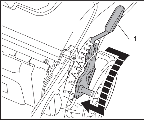
► 1. 修剪高度調整桿
