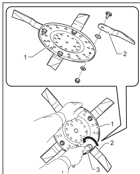
► 1. 基板 2. 修剪機刀片 3. 套筒扳手
