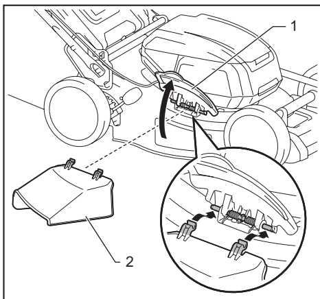
► 1. 右側蓋 2. 洩放組件
