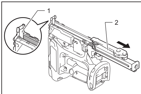
► 1. 縫隙 2. 副針槽
