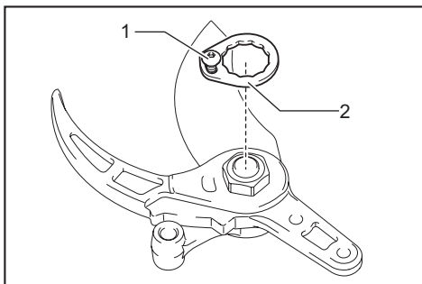
► 1. 板固定螺栓 2. 鎖定板
