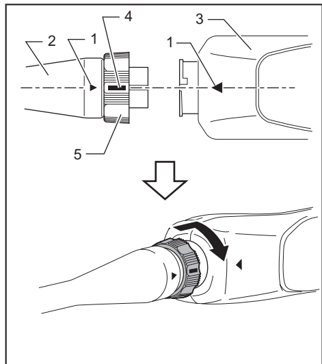
► 1. 三角標記 2. 連接電纜 3. 果樹剪 4. 耦合器上的標記 5. 耦合器
