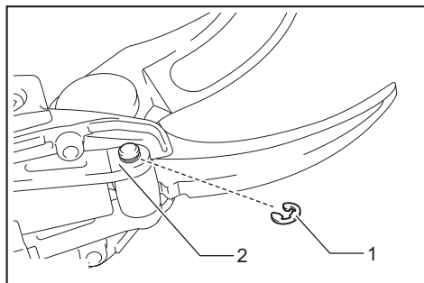
► 1. E型環 2. 連杆臂
