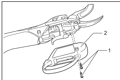
► 1. 螺栓 2. 扳機護環
