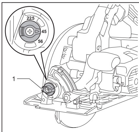
► 1. 主動止動器
