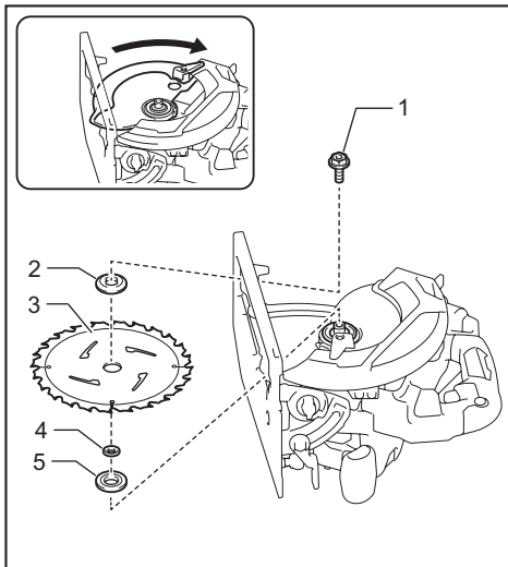
► 1. 六角螺栓 2. 外法蘭盤 3. 圓鋸機鋸片 4. 擋圈 5. 內法蘭盤
