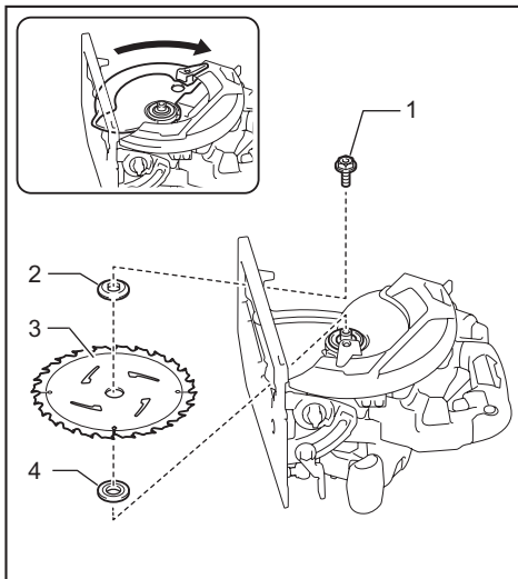
► 1. 六角螺栓 2. 外法蘭盤 3. 圓鋸機鋸片 4. 內法蘭盤
