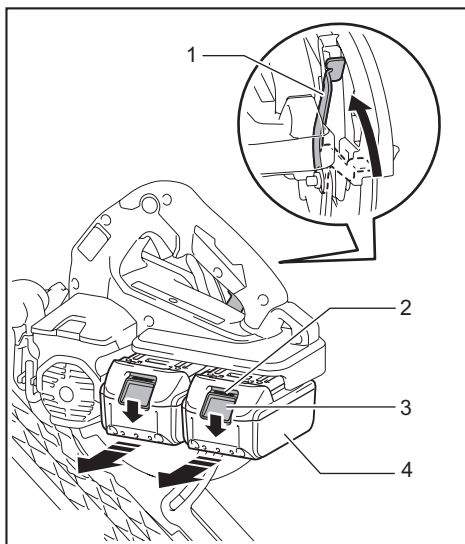
► 1. 調節鎖定桿 2. 紅色指示燈 3. 按鈕 4. 電池組
