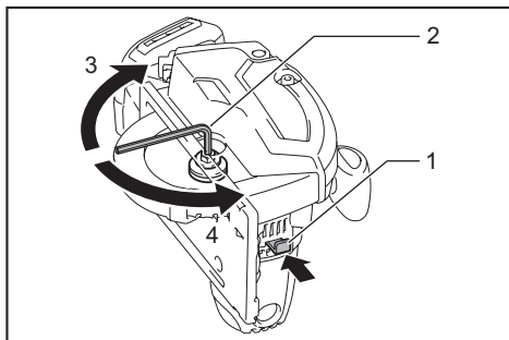
▶ 1. 軸鎖 2. 六角扳手 3. 擰緊 4. 旋鬆
