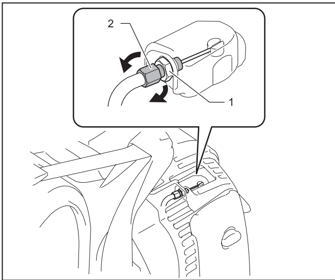
► 1. 固定螺帽 2. 纜線調整螺栓
