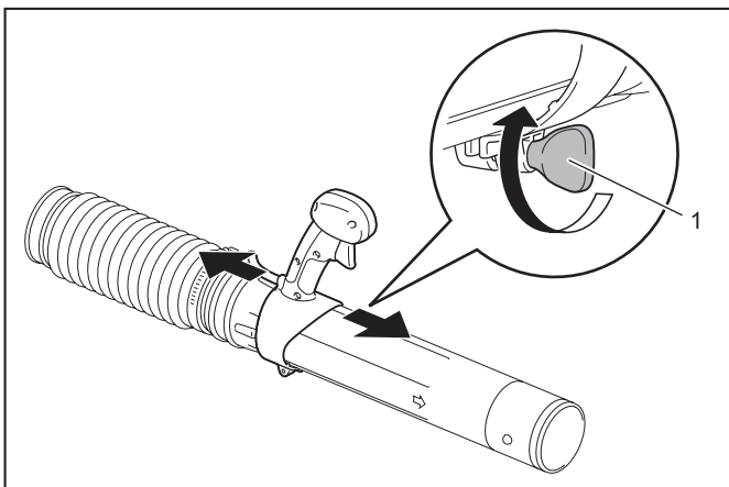
► 1. 螺絲
