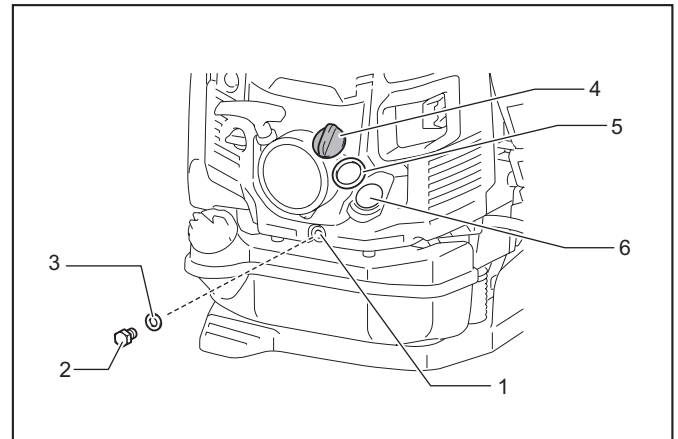
► 1. 排放孔 2. 排油螺栓 3. 襯墊 (鋁質墊片) 4. 機油蓋 5. 機油蓋襯墊 6. 機油孔
