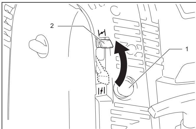
► 1. 起動注給泵 2. 阻風拉桿
