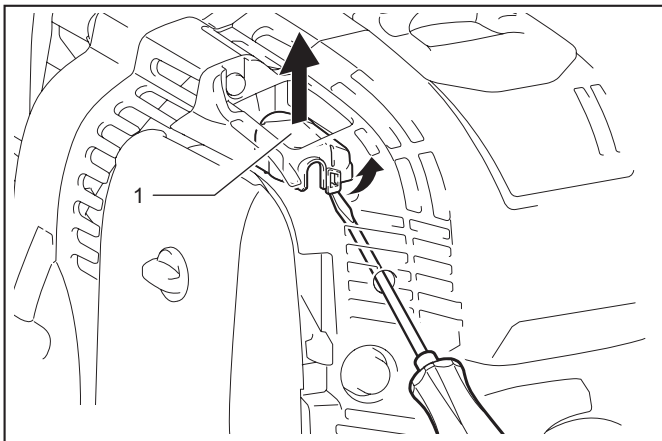
► 1. 化油器護蓋
