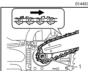
1. 鏈輪
