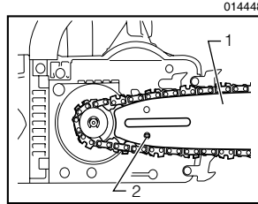
1. 導板 2. 孔
