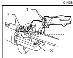
1. 掛鉤 2. 孔 3. 銷
