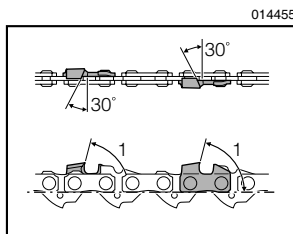
1. 側片角
