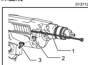
1. 深度規 2. 墊圈 3. 夾緊螺絲
