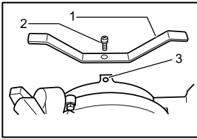
1. 輔助板 2. 螺絲 3. 基座
