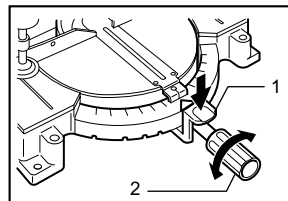
1. 鎖桿 2. 手柄
