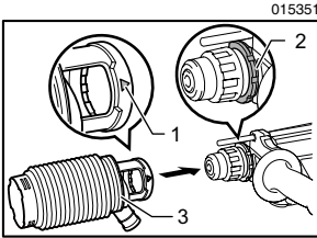
1. △符號 2. 凹槽 3. 防塵罩
