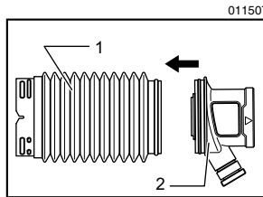
1. 風箱 2. 裝置
