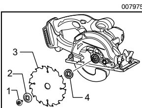
1. 六角螺絲 2. 外法蘭盤 3. 鋸片 4. 內法蘭盤
