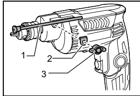
1. 深度規 2. 墊圈 3. 夾緊螺絲
