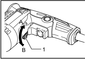
1. 反轉開關
