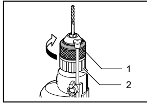
1. 套筒 2. 擋圈
