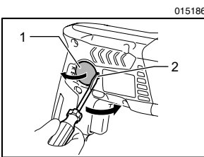
1. 碳刷夾蓋板 2. 凹槽部分
