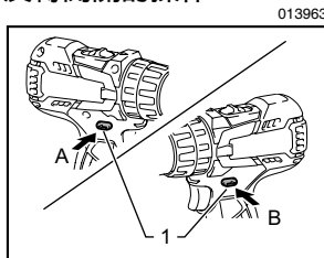
1. 反轉開關桿
