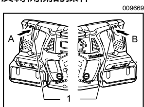
1. 反轉開關桿
