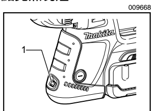
1. 照明燈
